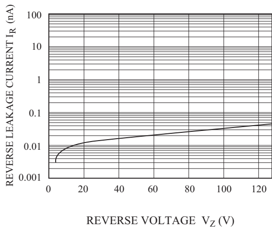
I_R - V_R
