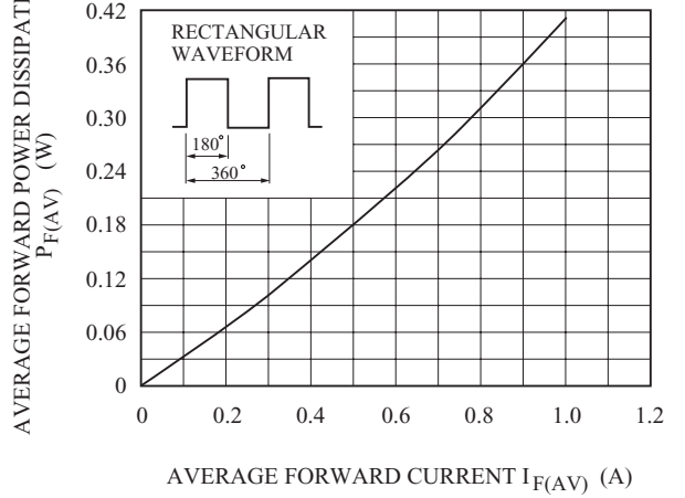
P_{F(AV)} - I_{F(AV)}
