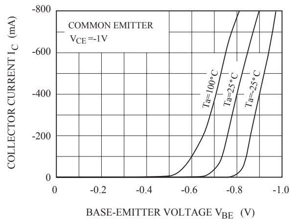
I_C - V_{BE}
