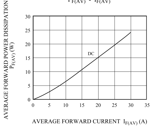
P_{F(AV)} - I_{F(AV)}
