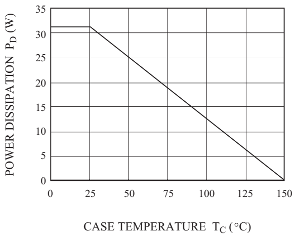
P_D - T_C
