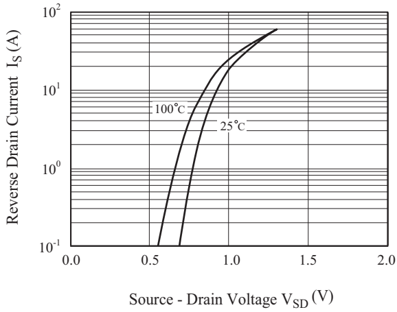
Fig7. I_S - V_{SD}
