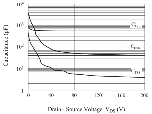
Fig 8. C - V_{DS}
