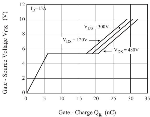
Fig9. Q_g - V_{GS}
