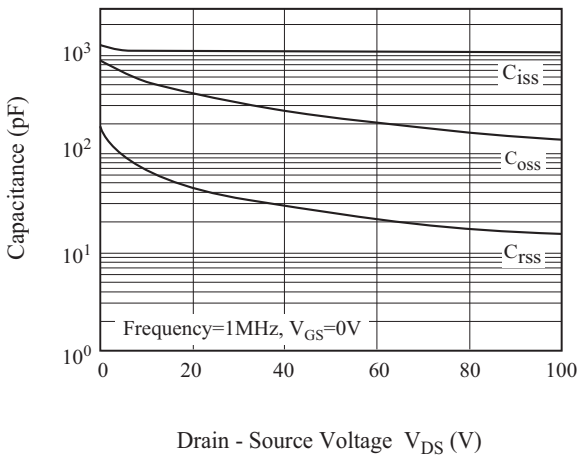
Fig 9. C - V_{DS}
