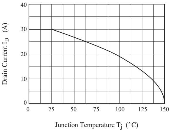
Fig11. I_D - T_j
