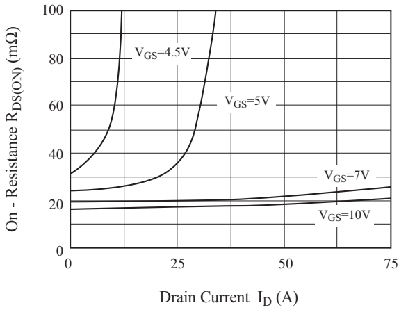
Fig7. R_{DS(ON)} - I_D
