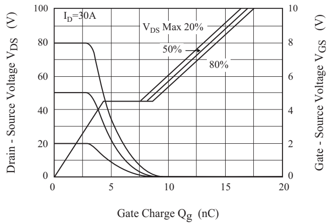
Fig10. Q_g - V_{GS}
