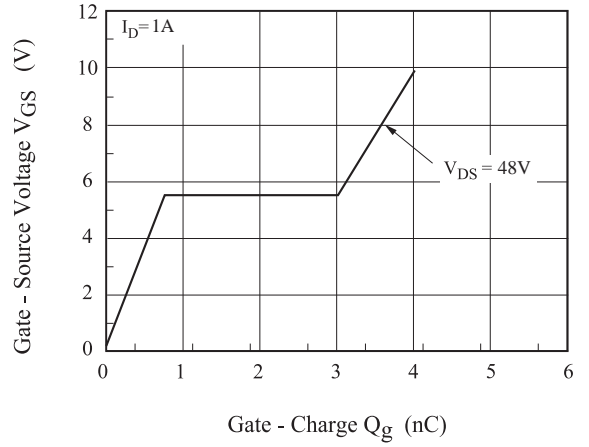
Fig8. V GS - Q g
