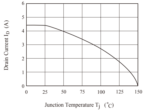
Fig10. I_D - T_j
