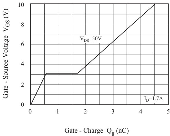
Fig9. Q_g - V_{GS}
