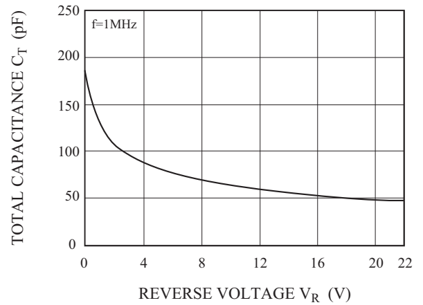
C_T - V_R
