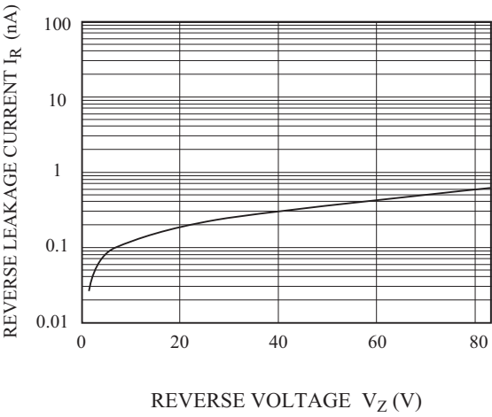
I_R - V_R
