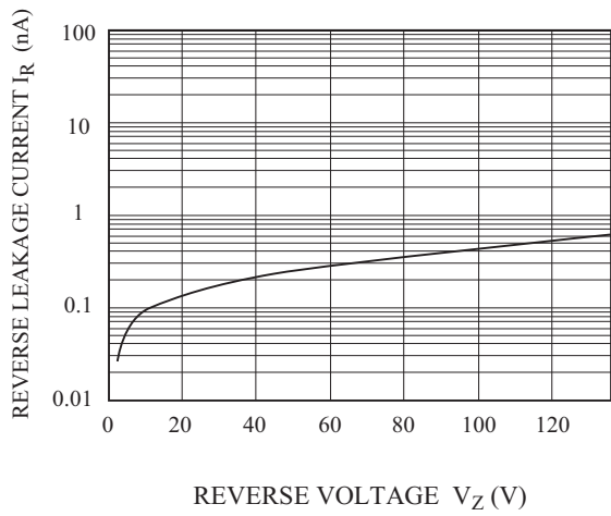
I_R - V_R
