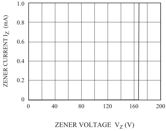
I_Z - V_Z
