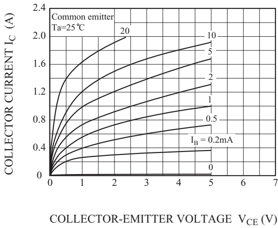
I_C - V_{CE}
