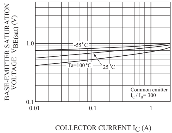
V_{BE(sat)} - I_C
