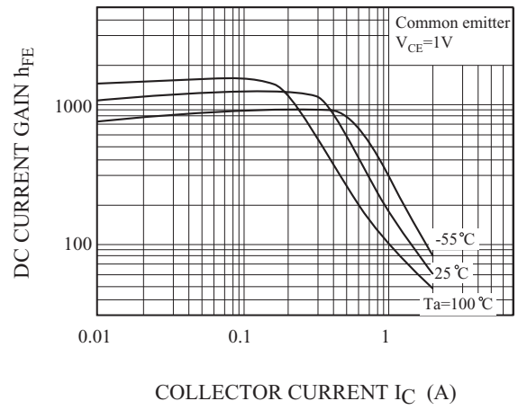
h_{FE} - I_C
