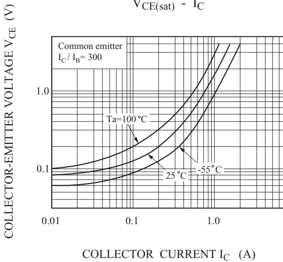
V_{CE(sat)} - I_C
