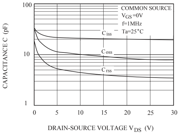
Fig 7. C - V DS
