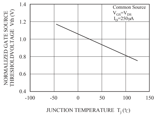
Fig 4. V_{th} - T_j
