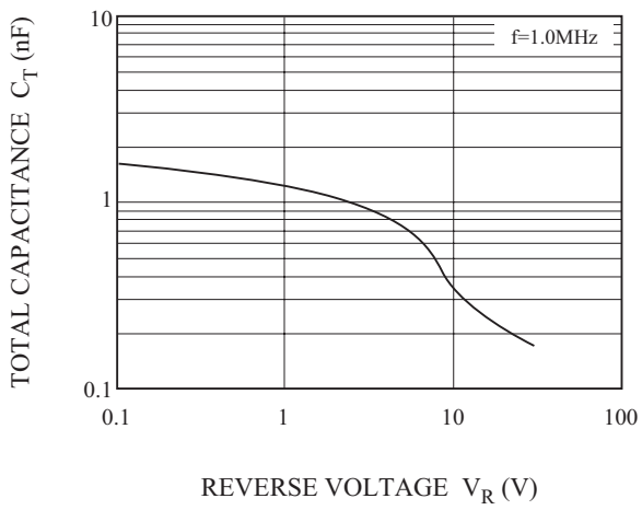
C_T - V_R
