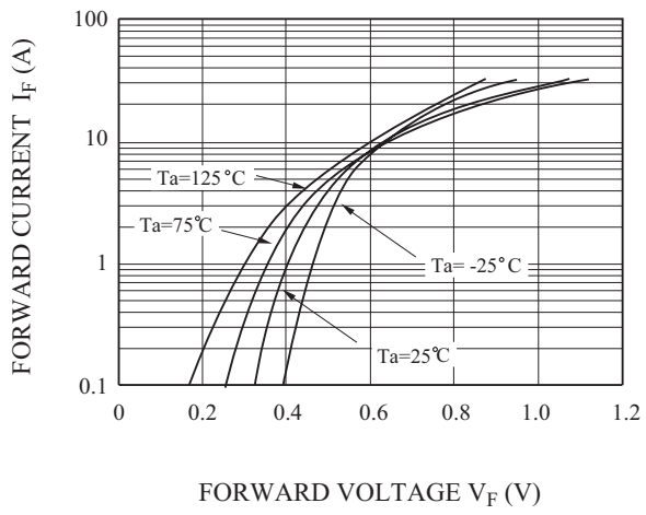
I_F - V_F
