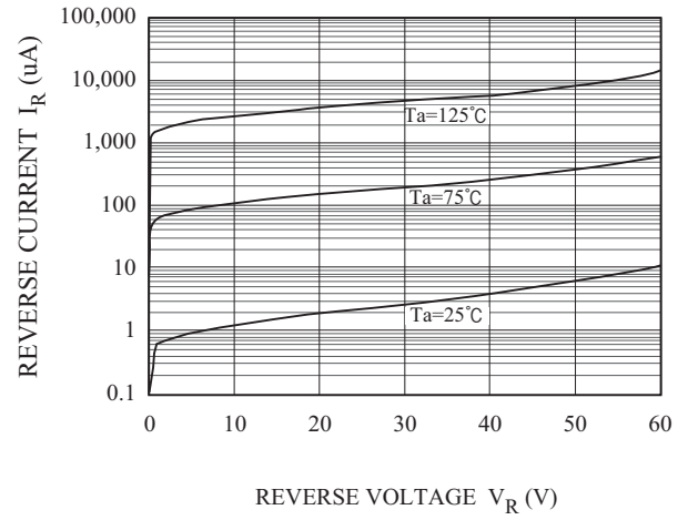
I_R - V_R
