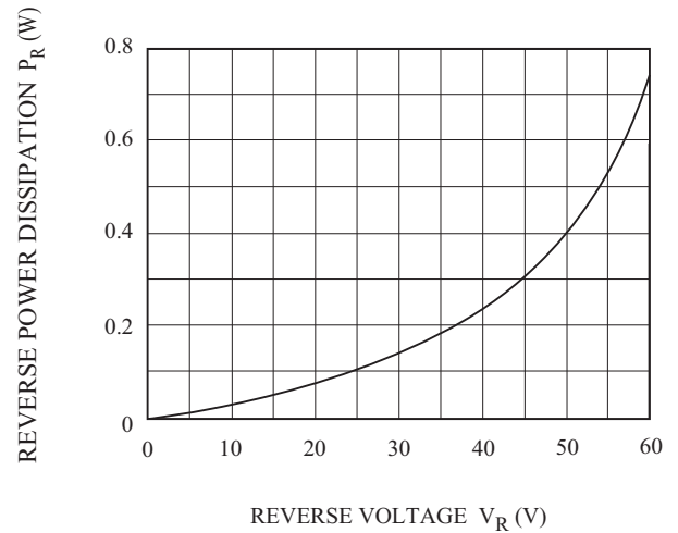
P_R - V_R
