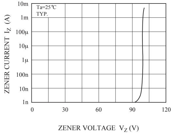
I_Z - V_Z
