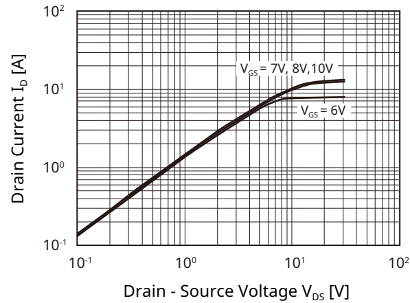
Fig 2. I_D - V_{DS} - 2
