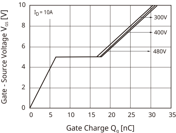
Fig 12. Q_g - V_{GS}
