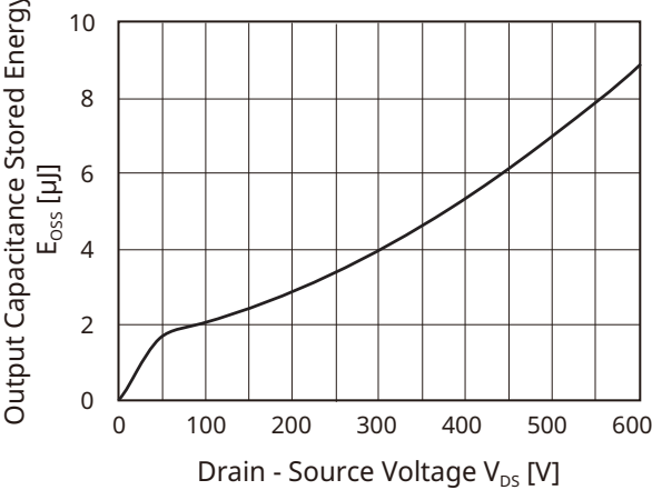
Fig 11. E_{OSS} - V_{DS}
