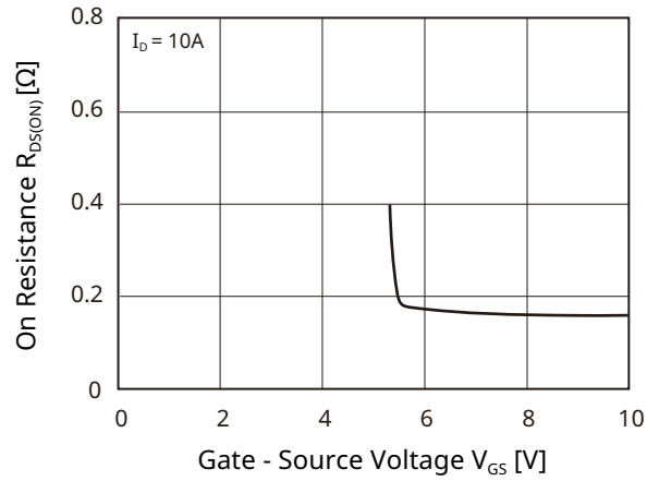
Fig 5. R_{DS(ON)} - V_{GS}
