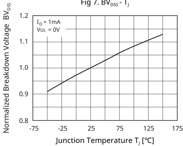
Fig 7. BV_{DSS} - T_J
