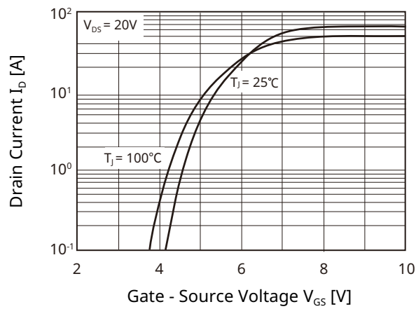
Fig 3. I_D - V_{GS}
