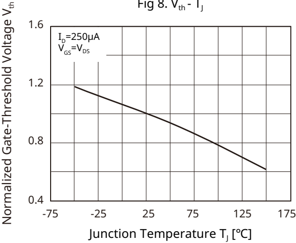
Fig 8. V_{th} - T_J
