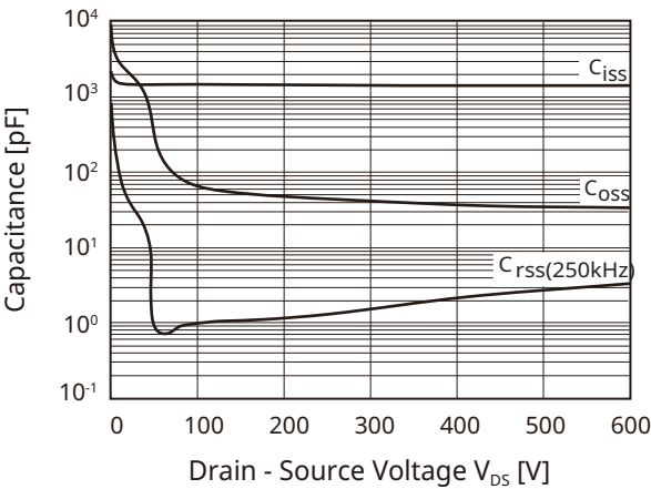
Fig 10. Capacitance V_{DS}
