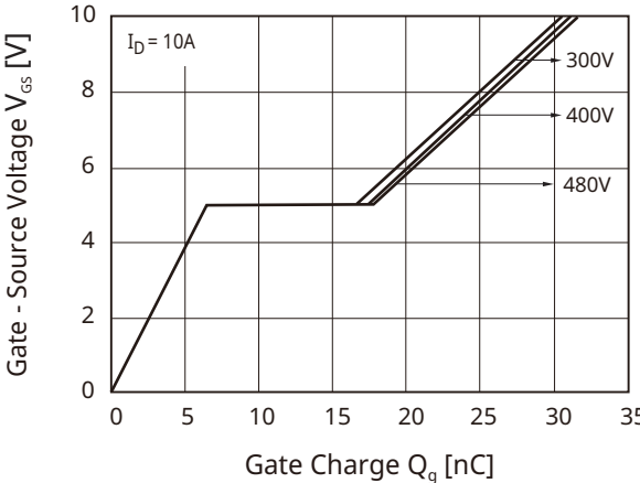
Fig 12. Q_g - V_{GS}
