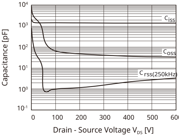
Fig 10. Capacitance V_{DS}
