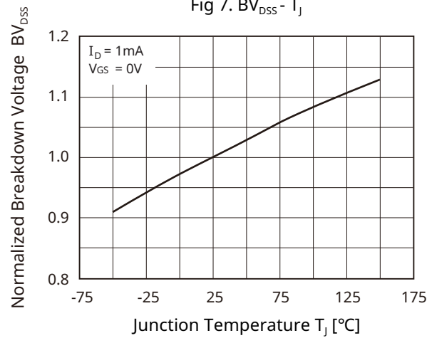
Fig 7. BV_{DSS} - T_J
