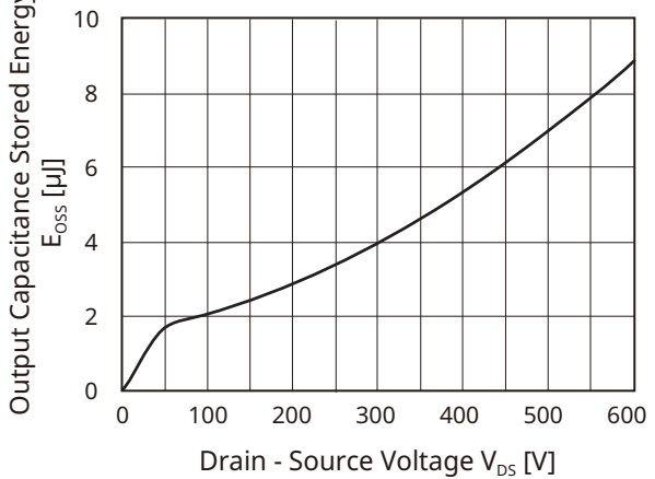
Fig 11. E_{OSS} - V_{DS}
