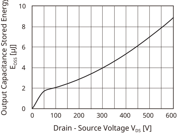
Fig 11. E_{OSS} - V_{DS}
