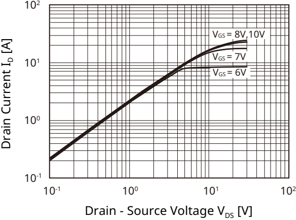
Fig1. I_D - V_{DS} - 2
