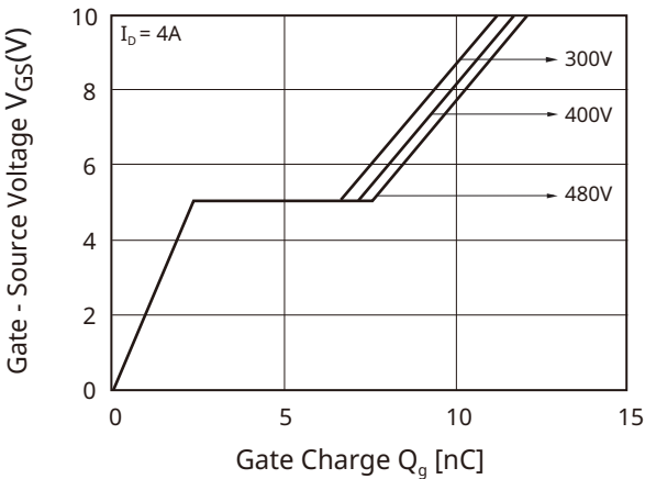
Fig11. Q_g - V_{GS}
