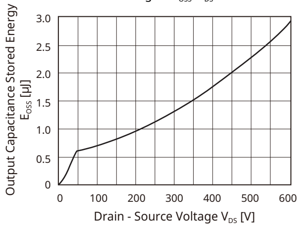
Fig11. E_{oss} - V_{DS}
