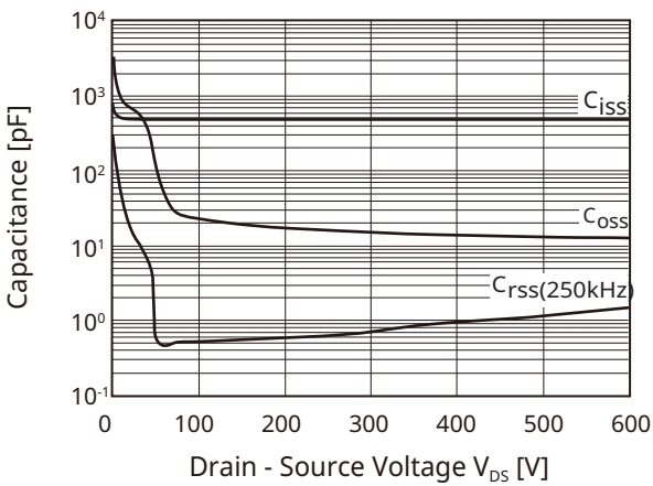
Fig10. Capacitance V_{DS}
