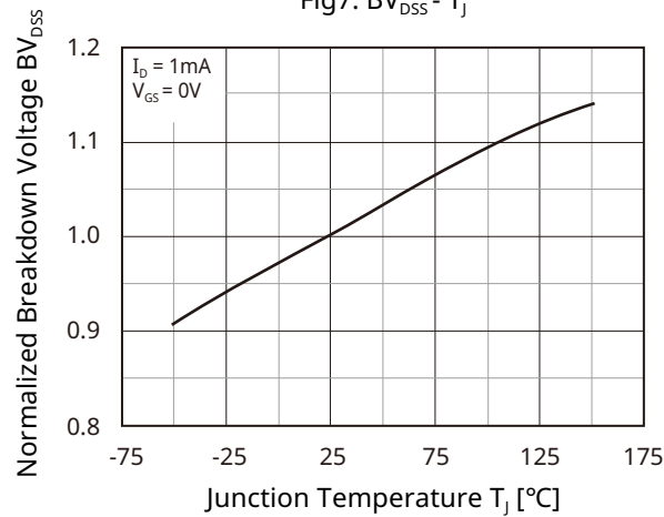
Fig7. BV_{DSS} - T_J
