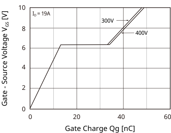
Fig12. Q_g - V_{GS}
