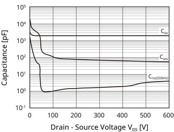
Fig10. Capacitance - V_{DS}
