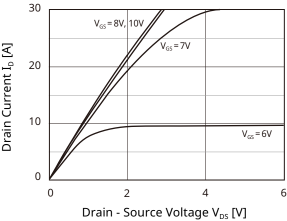
Fig1. I_D - V_{DS} -1
