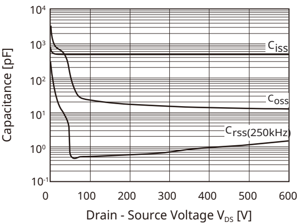
Fig10. Capacitance V_{DS}
