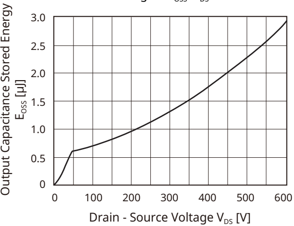
Fig11. E_{OSS} - V_{DS}
