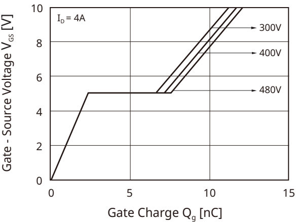
Fig11. Q_g - V_{GS}
