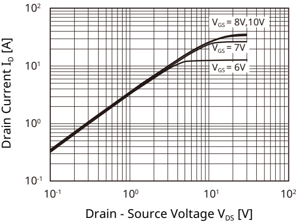
Fig1. I_D - V_{DS} - 2
