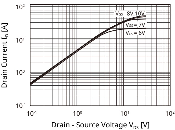
Fig1. I_D - V_{DS} - 2
