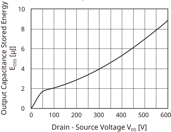
Fig 11. E_{OSS} - V_{DS}
