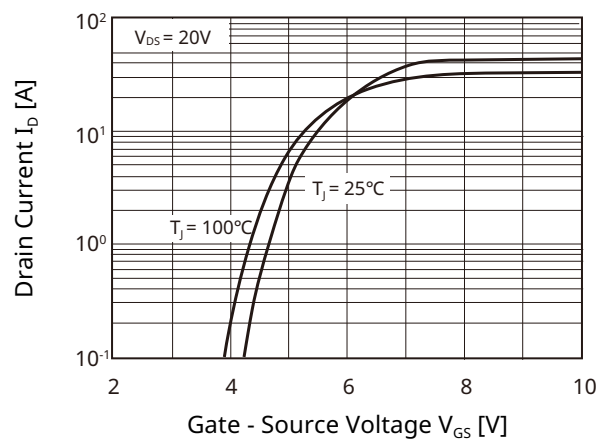
Fig3. I_D - V_{GS}
