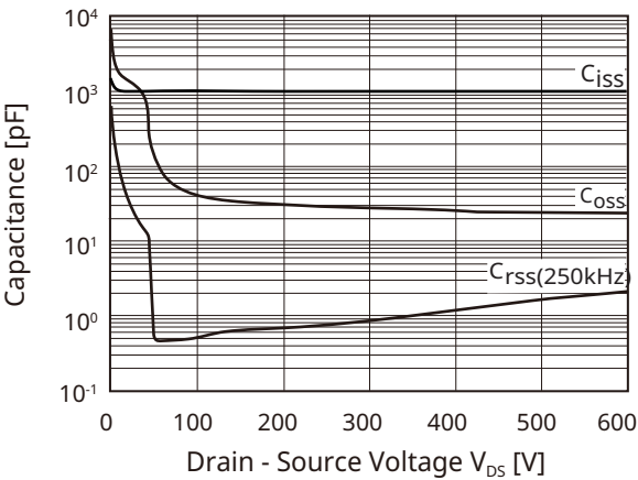
Fig10. Capacitance V_{DS}
