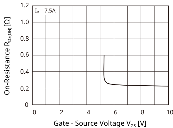
Fig5. R_{DS(ON)} - V_{GS}
