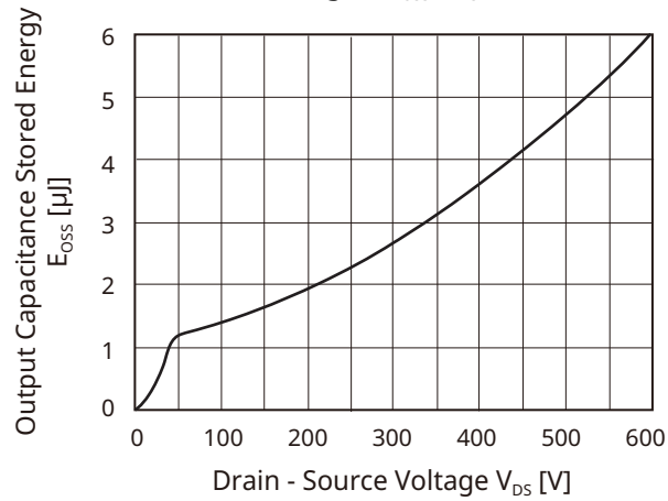
Fig11. E_{OSS} - V_{DS}
