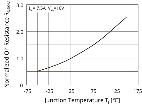
Fig6. R_{DS(ON)} - T_J
