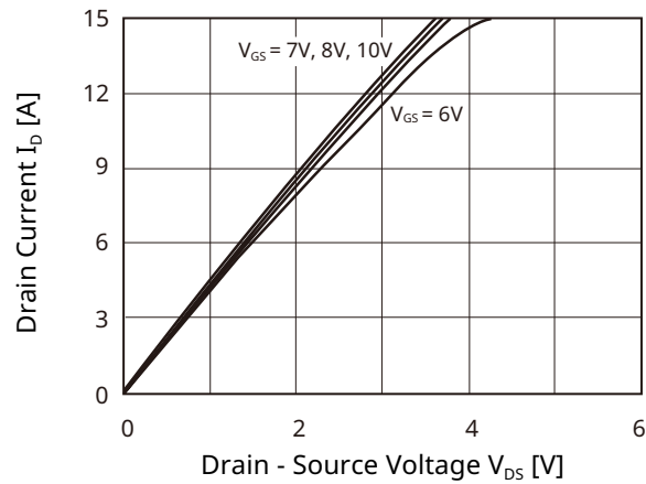
Fig1. I_D - V_{DS} - 1
