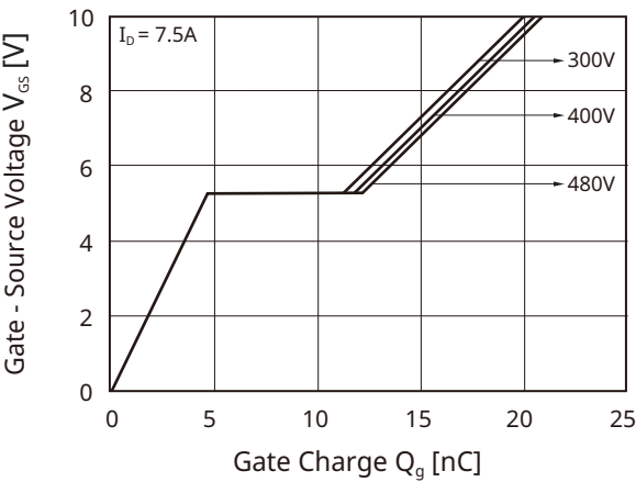
Fig11. Q_g - V_{GS}
