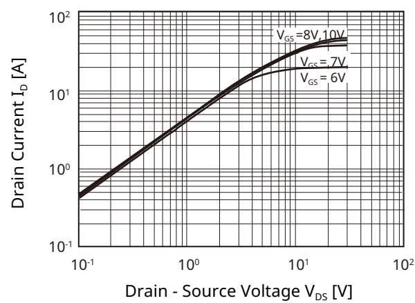
Fig1. I_D - V_{DS} - 2
