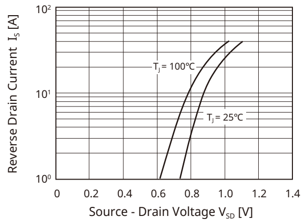
Fig9. I_S - V_{SD}
