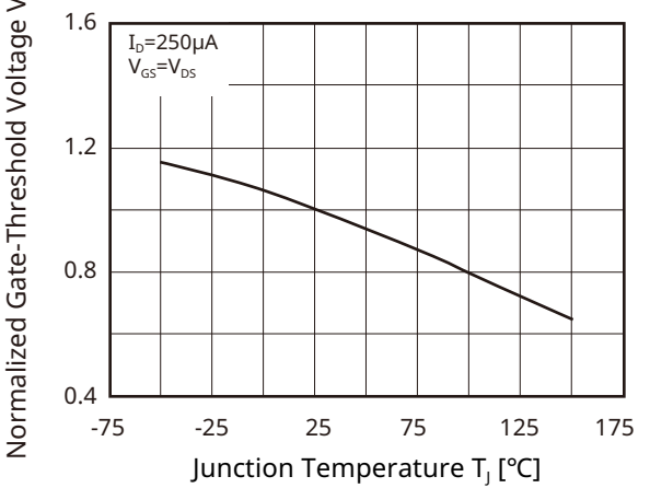
Fig 8. V_{th} - T_J
