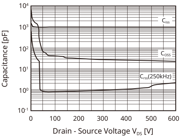
Fig 10. Capacitance V_{DS}
