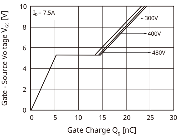
Fig 12. Q_g - V_{GS}
