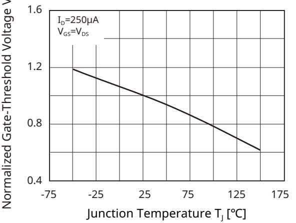
Fig 8. V_{th} - T_J
