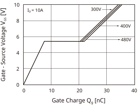
Fig 12. Q_g - V_{GS}
