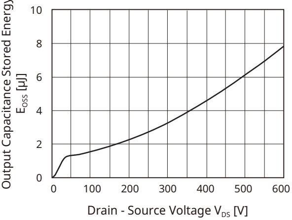
Fig 11. E_{OSS} - V_{DS}
