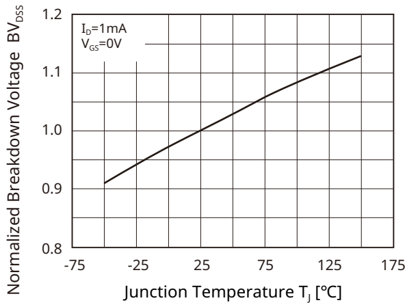
Fig 7. BV_{DSS} - T_J
