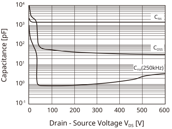
Fig 10. Capacitance V_{DS}
