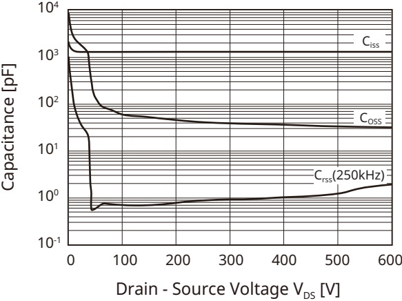
Fig 10. Capacitance V_{DS}
