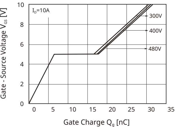
Fig 12. Q_g - V_{GS}
