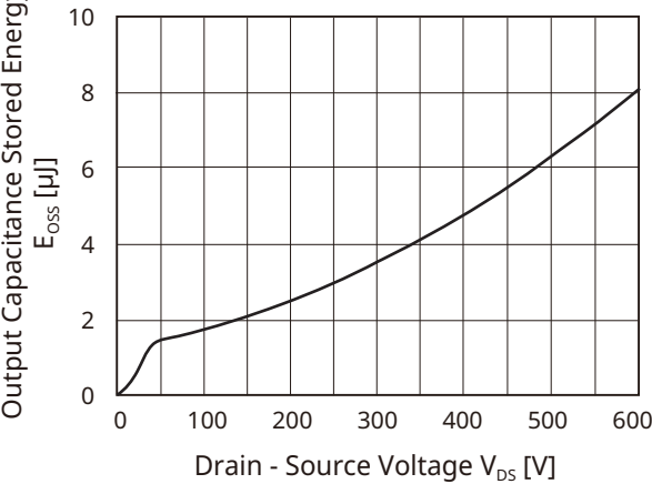
Fig 11. E_{OSS} - V_{DS}
