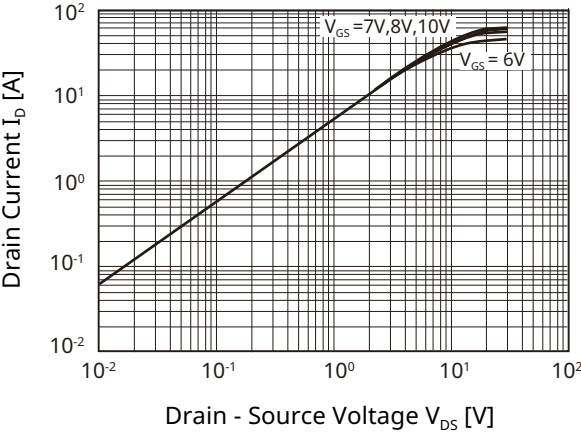
Fig 2. I_D - V_{DS} - 2
