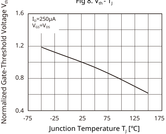
Fig 8. V_{th} - T_J
