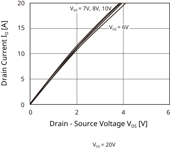
Fig 1. I_D - V_{DS} - 1
