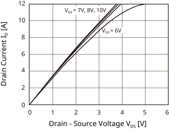
Fig 1. I_D - V_{DS} - 1
