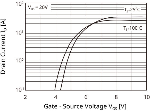
Fig 3. I_D - V_{GS}
