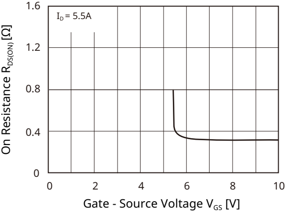
Fig 5. R_{DS(ON)} - V_{GS}
