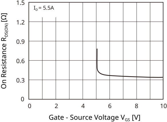
Fig 5. R_{DS(ON)} - V_{GS}
