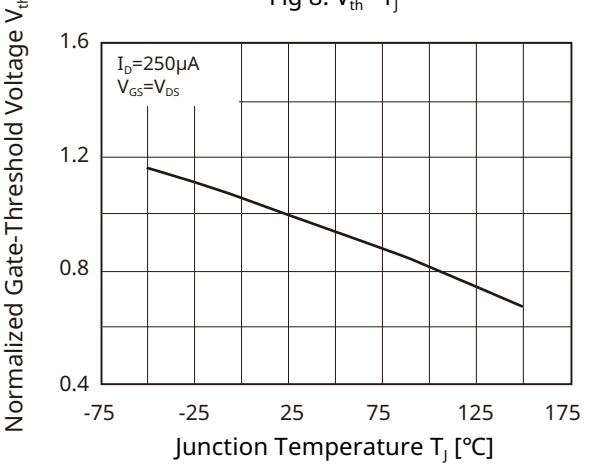
Fig 8. V_{th} - T_J
