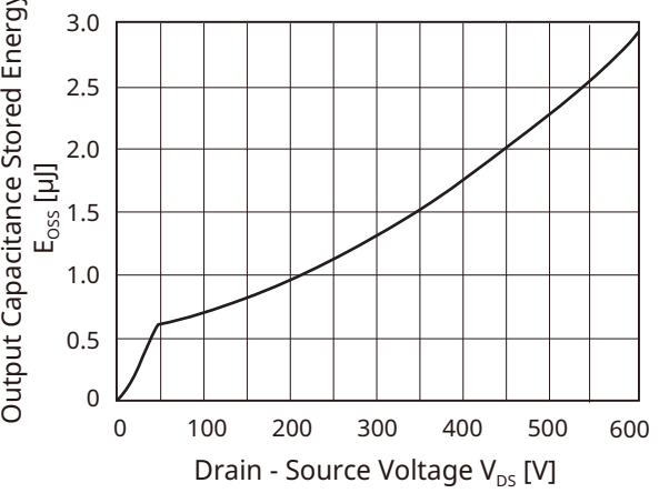
Fig 11. E_{OSS} - V_{DS}
