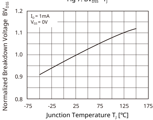
Fig 7. BV_{DSS} - T_J
