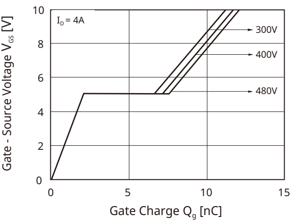
Fig 12. Q_g - V_{GS}
