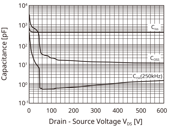
Fig 10. Capacitance V_{DS}
