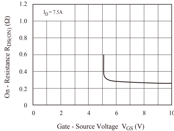
Fig5. R_{DS(ON)} - V_{GS}
