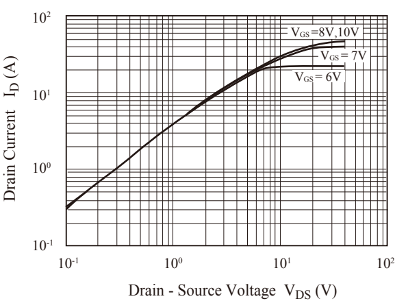
Fig2. I_D - V_{DS} - 2
