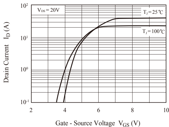
Fig3. I_D - V_{GS}
