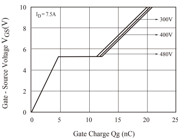
Fig12. Q_g - V_{GS}
