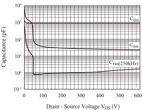
Fig10. Capacitance - V_{DS}
