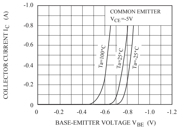
I_C - V_{BE}
