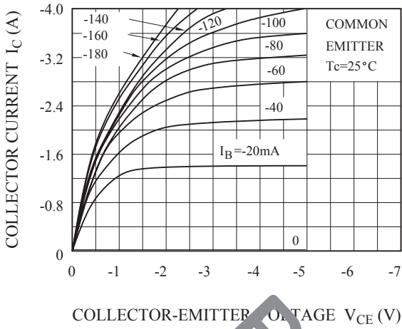
I_C - V_{CE}
