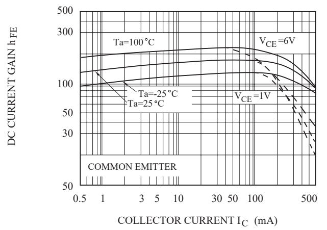
h_{FE} - I_C
