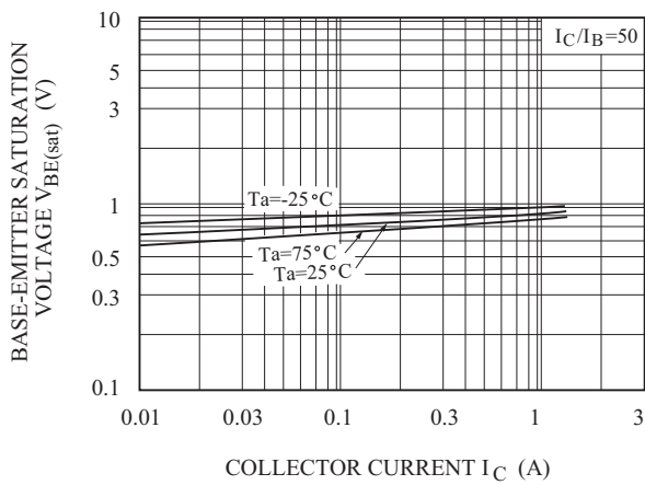
V_{BE(sat)} - I_C
