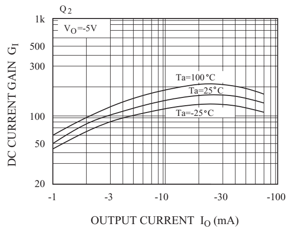
G_I - I_O
