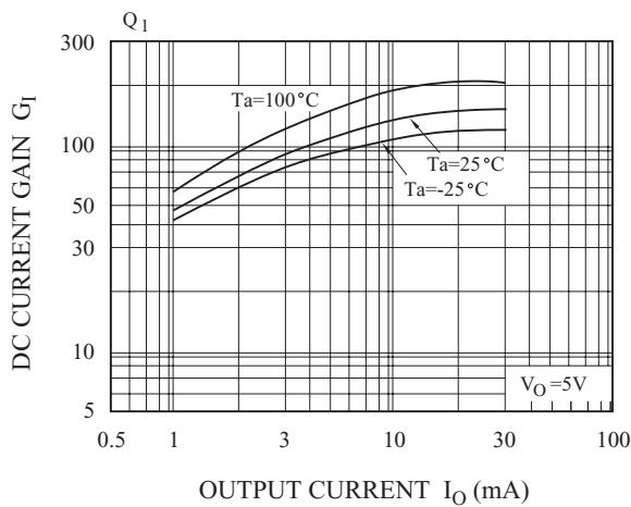
G_I - I_O
