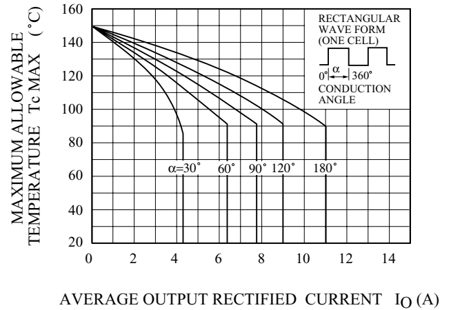
T_c - I_O
