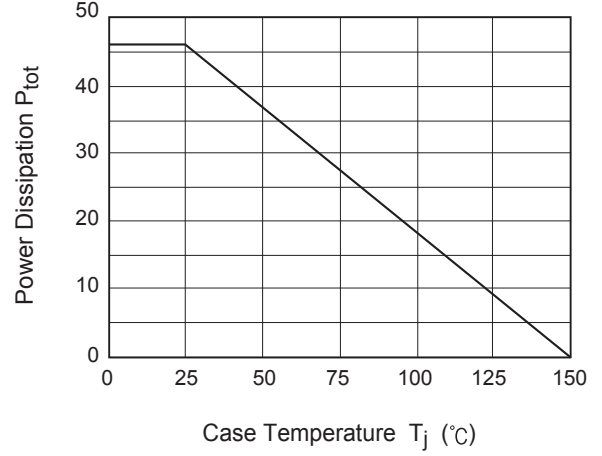
Fig 14. P_{tot} - T_C
