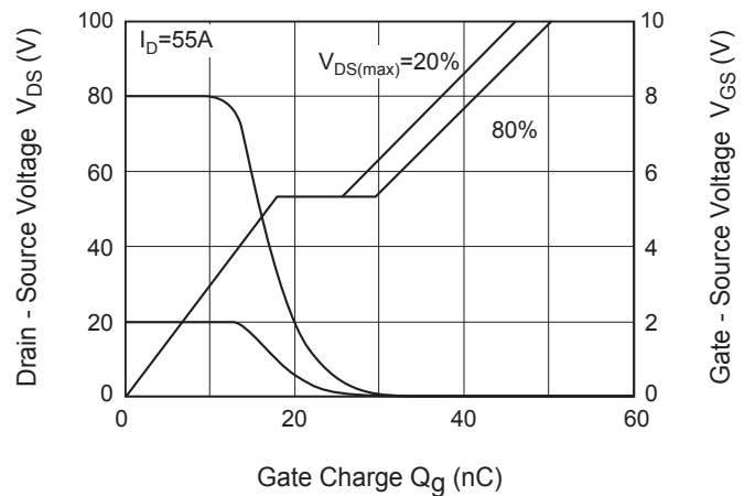
Fig12. Q_g - V_{DS}
