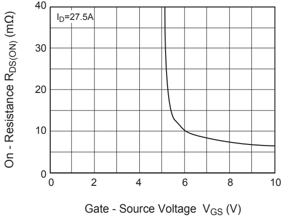
Fig5. R_{DS(ON)} - V_{GS}
