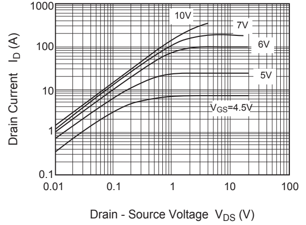
Fig2. I_D - V_{DS} - II
