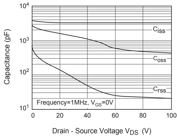
Fig 11. C - V_{DS}
