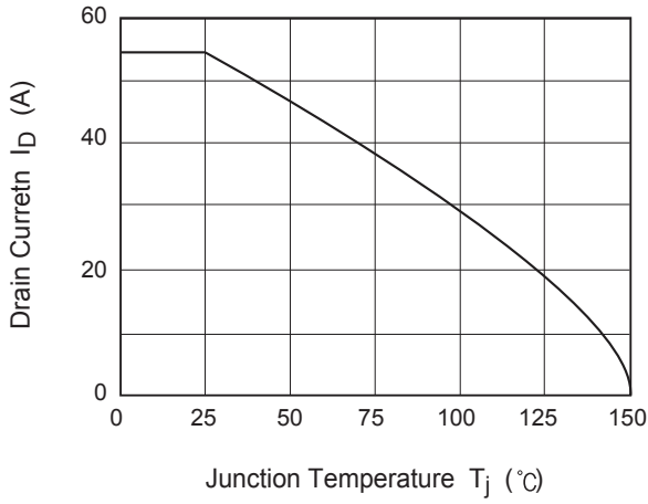
Fig13. I_D - T_j
