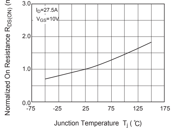
Fig6. R_{DS(ON)} - T_j
