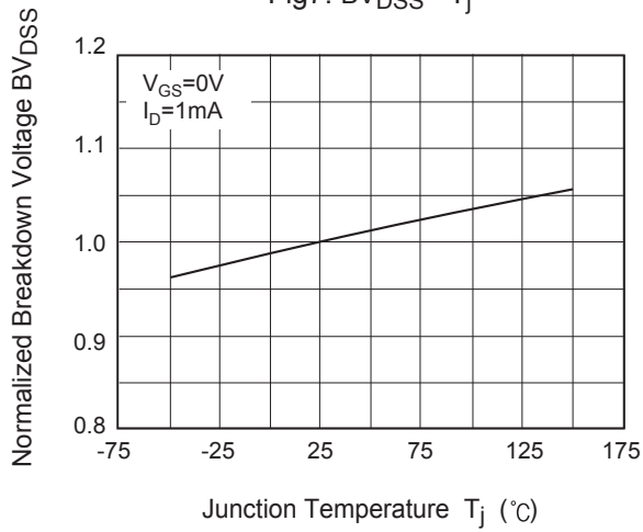
Fig7. BV_{DSS} - T_j
