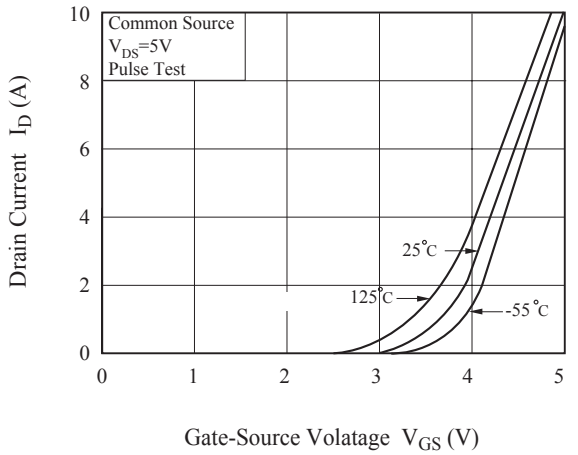
Fig3. I_D - V_{GS}
