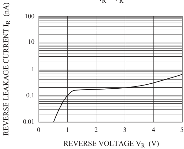
I_R - V_R
