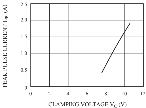
I_{PP} - V_C
