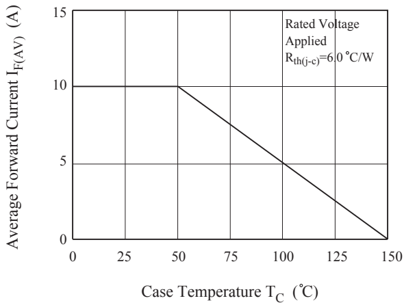
I_{F(AV)} - T_C
