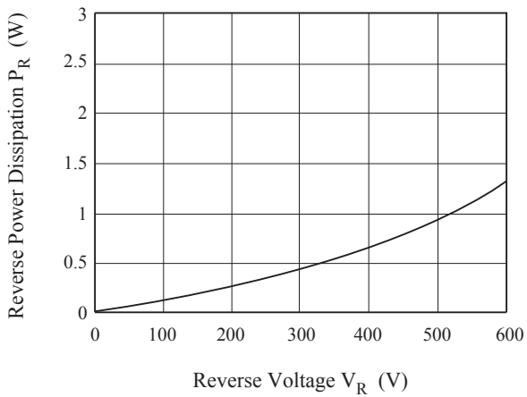
P_R - V_R
