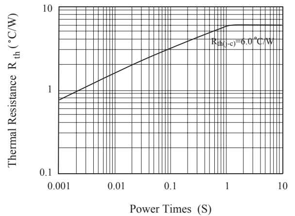
R_{th(j-c)}
