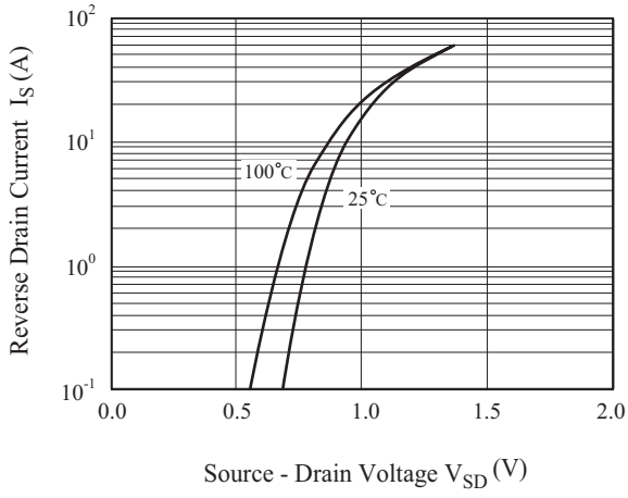
Fig7. I_S - V_{SD}
