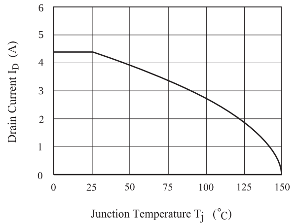
Fig10. I_D - T_j
